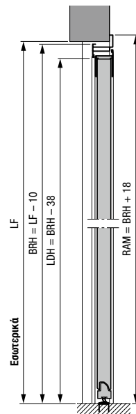
Πλαϊνή πόρτα με γωνιακή κάσα αλουμινίου προφίλ τύπου 2 Άνοιγμα προς τα έξω
