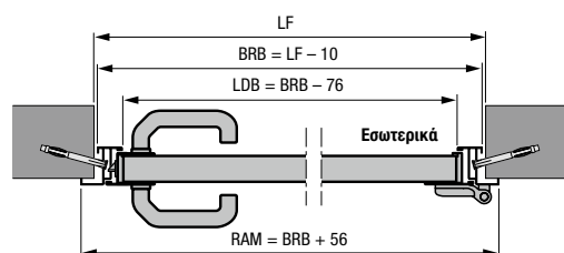
Πλαϊνή πόρτα με γωνιακή κάσα αλουμινίου προφίλ τύπου 1 ή 2 Άνοιγμα προς τα μέσα
