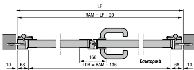
Δίφυλλη πλαϊνή πόρτα με απλή κάσα αλουμινίου προφίλ τύπου 2 Τοποθέτηση στο άνοιγμα
