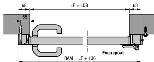
Πλαϊνή πόρτα με απλή κάσα αλουμινίου προφίλ τύπου 1 Τοποθέτηση πίσω από το άνοιγμα
