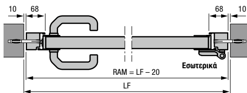
Πλαϊνή πόρτα με απλή κάσα αλουμινίου προφίλ τύπου 2 Τοποθέτηση στο άνοιγμα
