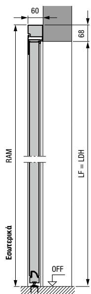
Πλαϊνή πόρτα με απλή κάσα αλουμινίου προφίλ τύπου 2 Τοποθέτηση πίσω από το άνοιγμα
