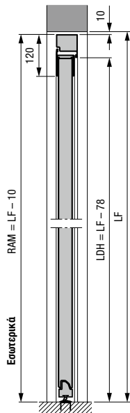
Πλαϊνή πόρτα με απλή κάσα αλουμινίου προφίλ τύπου 2 Τοποθέτηση στο άνοιγμα
