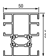
Προφίλ επέκτασης 50 mm
